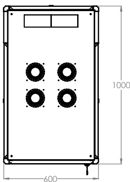
ВИД СВЕРХУ
