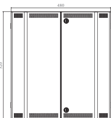
ВИД СПЕРЕДИ
