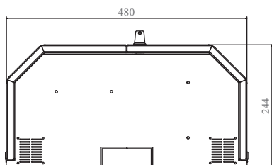
ВИД СНИЗУ
