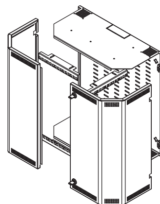
ДЕТАЛЬНЫЙ ВИД
